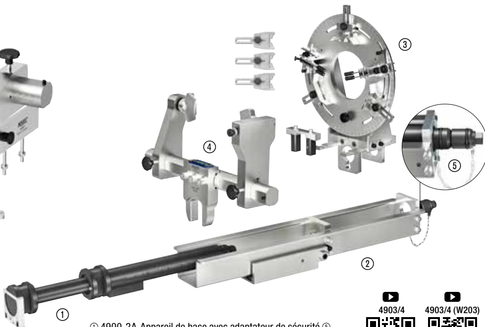
Réglage vertical, actionnement horizontal. Orientable !
