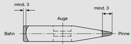
Schematischer Verlauf der Härtezone
